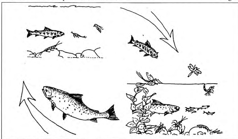
Schematisk bild över öringens vandring mellan rinnande vatten och sjö. Örings- ynglet kläcks på försommaren i t ex en bäck, lever i bäcken under 2-3 år för att sedan vandra ned- eller uppströms till en sjö. I sjön tillväxer öringen under 1-3 år för att sedan återvända till bäcken den föddes i för att leka.
